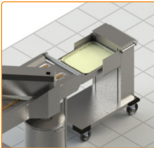
Chariot niveau constant Rampe à rouleaux 430 mm Cellule détectrice d'objet
