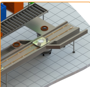
Goulotte humide longueur 800 mm de dévoiement "en S"
