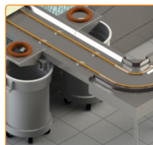
Convoyeur épaisseur spéciale 80 mm
